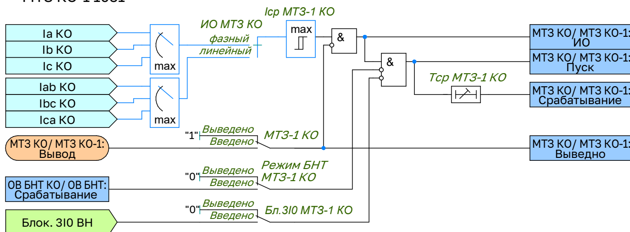
МТЗ КО-1 1031
