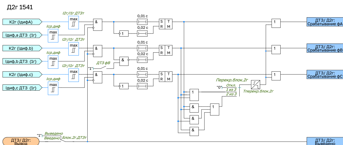
Рисунок 2.4 – Функциональная схема логики блокировки по второй гармонике
